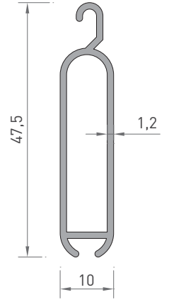
2217 FİTİLLİ ALT PARÇA 0.340 kg/mt
