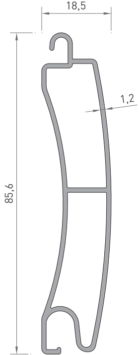
2213 PALET PROFİL 0.705 kg/mt
