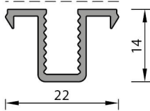
6 MM CAM ÇITA PROFİL V.ES.296 0.177 kg/mt
