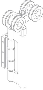
Rulmanlı üst menteşe roller top hinge
