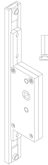
ispanyolet gövde espagnolette body
